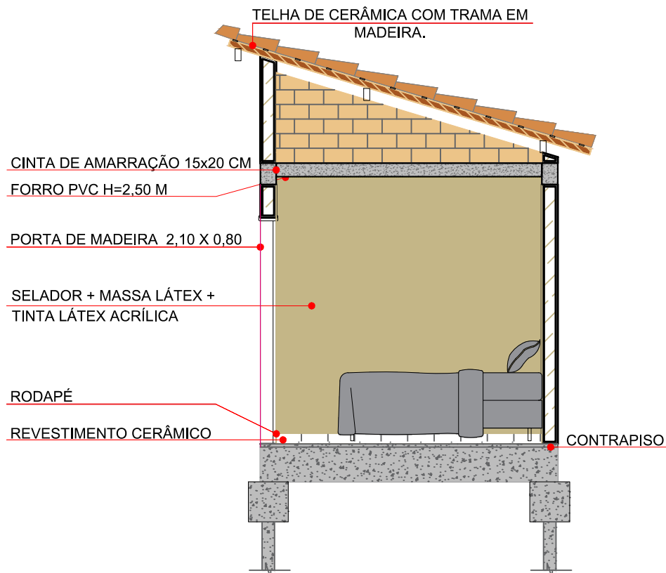
PROJETO CORTE ESC: 1:50
