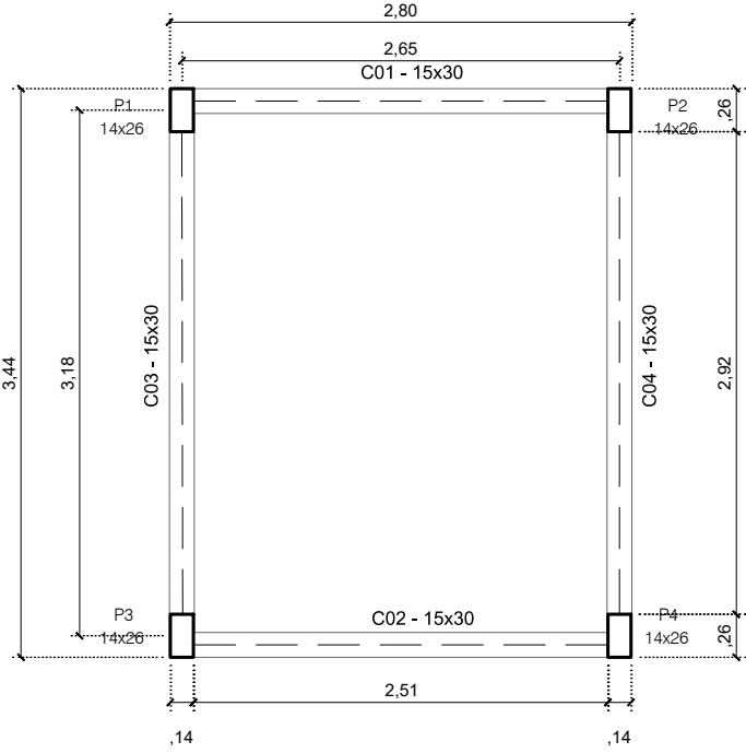
ESTRUTURA FORMA DA COBERTURA (NÍVEL 260cm) ESC: 1:50
