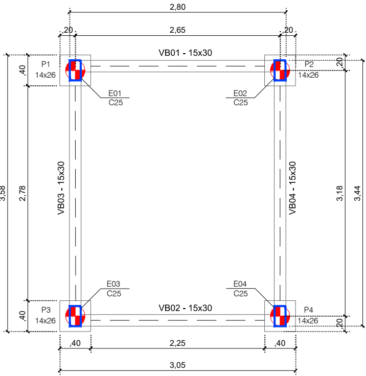
ESTRUTURA FORMA DA FUNDAÇÃO (NÍVEL -10cm) ESC: 1:50
