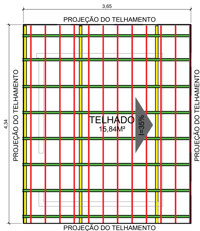
COBERTURA ESTRUTURA DA COBERTURA ESC: 1:50
