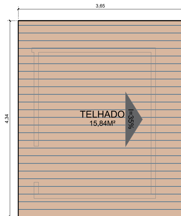
COBERTURA COBERTURA EM TELHA CERÂMICA ESC: 1:50
